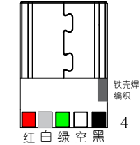
Micro usb母头焊接面
