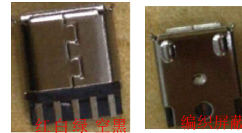
母头线束焊接实物图
